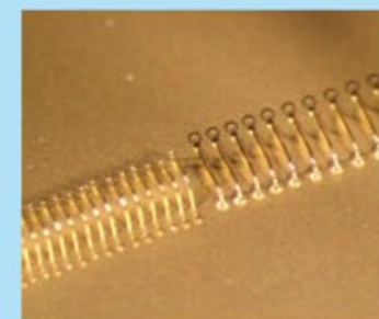
Wedge & ball bonds
